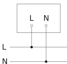
aansluitschema slave/draadloze masterkoppeling
